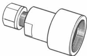
19.1.20501 Estrattore volano Flywheel puller
