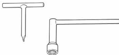
19.1.20522 Attrezzo per registrazione valvole Valve clearance adjustment tool
