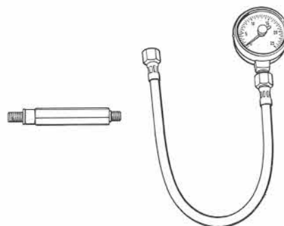
19.1.20524 Attrezzo per controllo compressione Compression check tool
