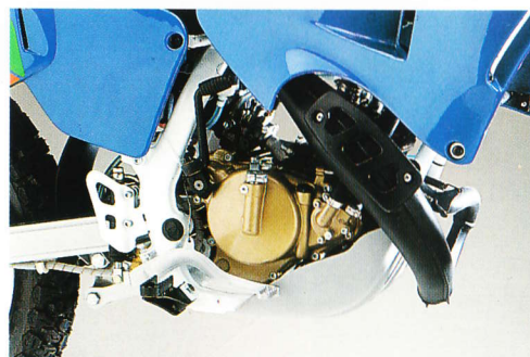
Vista laterale motore, scarico, paracoppa
