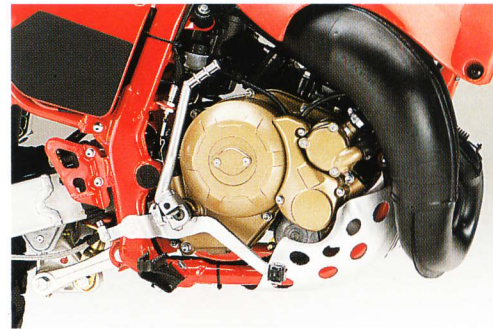
Vista laterale motore, scarico, paracoppa in alluminio
